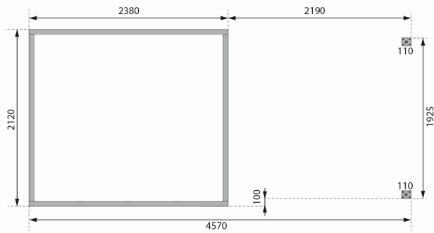
Fundamentplan mit Boden (in mm)
