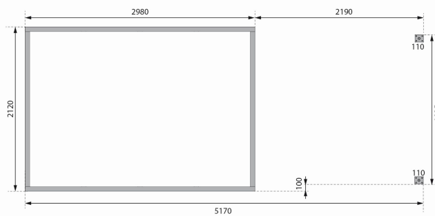
Fundamentplan ohne Boden (in mm)
