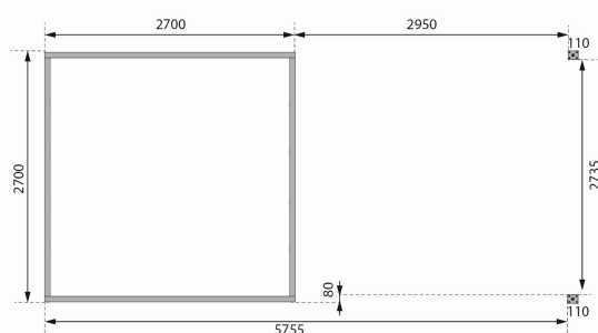
Fundamentplan ohne Boden (in mm)
