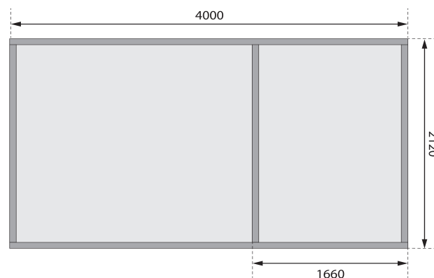
Fundamentplan ohne Boden (in mm)
