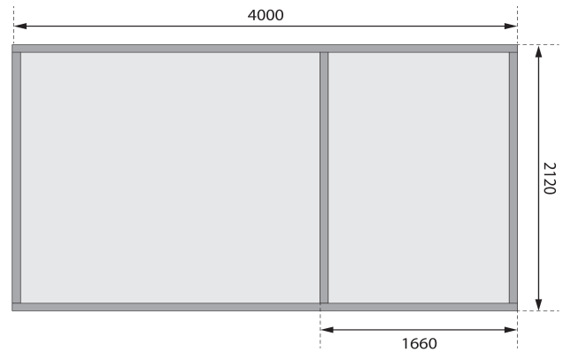
Fundamentplan ohne Boden (in mm)
