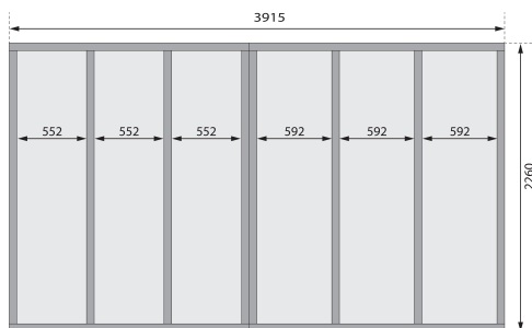
Fundamentplan mit Boden (in mm)
