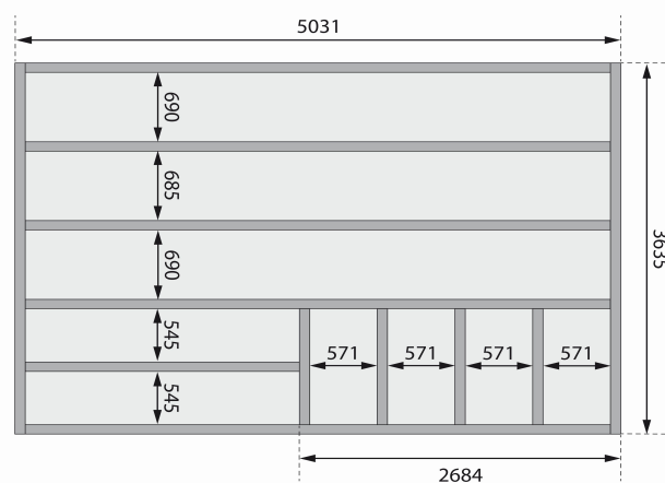
Fundamentplan mit Boden (in mm)
