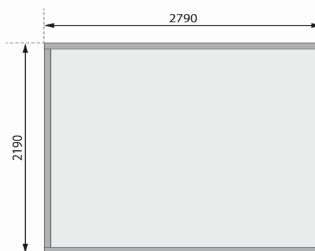
Fundamentplan ohne Boden (in mm)
