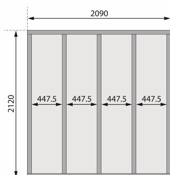
Fundamentplan mit Boden (in mm)
