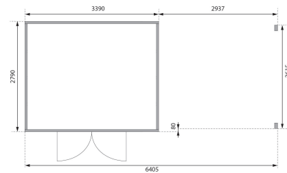
Fundamentplan ohne Boden (in mm)
