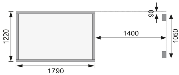
Fundamentplan ohne Boden (in mm)
