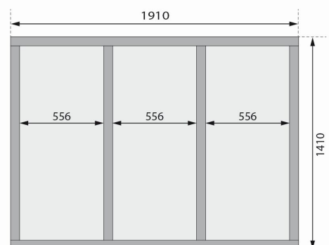
Fundamentplan mit Boden (in mm)
