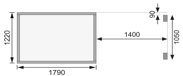
Fundamentplan ohne Boden (in mm)
