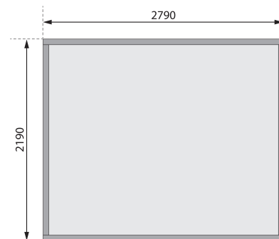
Fundamentplan ohne Boden (in mm)
