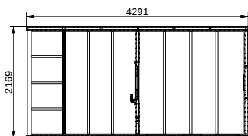
Grundriss
