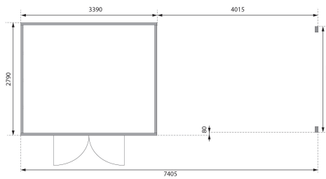
Fundamentplan ohne Boden (in mm)
