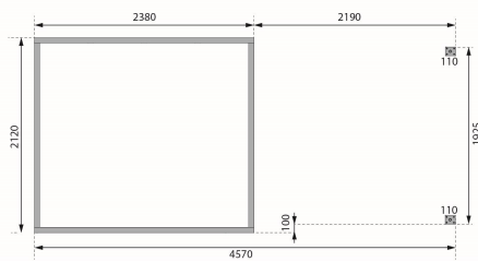
Fundamentplan ohne Boden (in mm)
