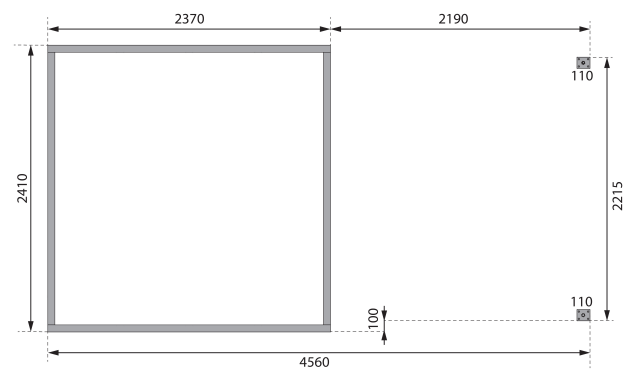
Fundamentplan ohne Boden (in mm)
