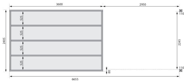
Fundamentplan mit Boden (in mm)
