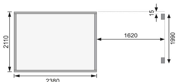
Fundamentplan ohne Boden (in mm)
