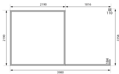
Fundamentplan ohne Boden (in mm)
